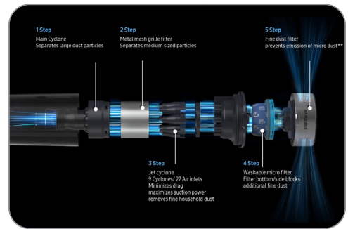
Système de filtration à cinq couches
